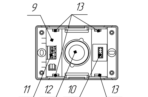
Рисунок 1.1 - Сигнализаторы оксида углерода и горючих газов СТГ-1. Внешний вид
