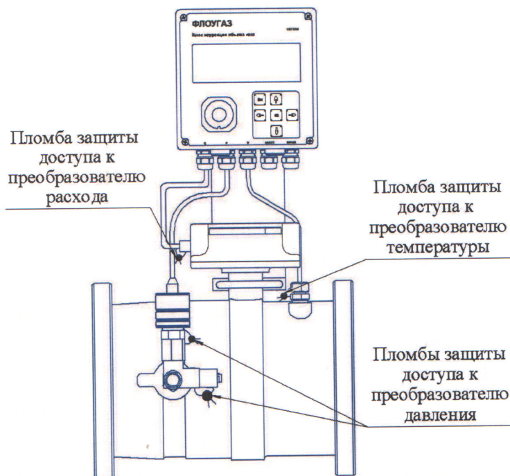
Рисунок 2 - Схема опломбировки комплекса
