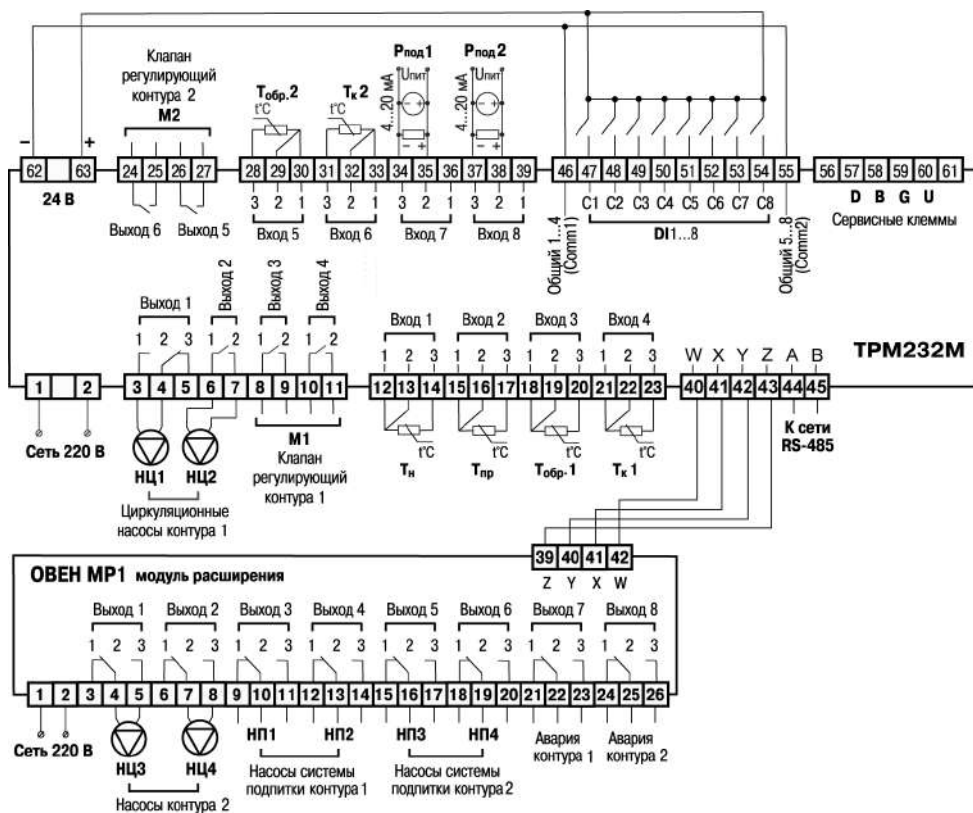
Рисунок 6.4 – Схема подключения для конфигурации № 4
