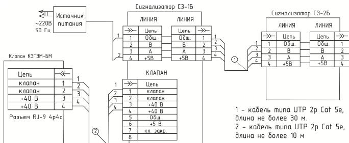
Рис. 6. – Система автономного контроля загазованности SGK-2-Б. Схема электрических соединений
