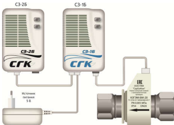
Рис. 5. – Система автономного контроля загазованности SGK-2-Б.
