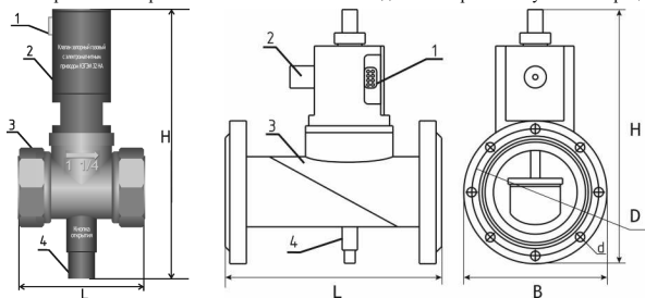
Рисунок 3. – Клапан КЗГЭМ.
