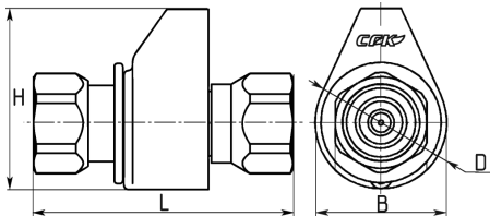
Рисунок 4. – Габаритные размеры клапана КЗГЭМ-Б.
