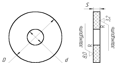
Материал: Пластина ТКМЦ-М-2 ГОСТ 7338-90 Рисунок Б.1 – Уплотнительная шайба
