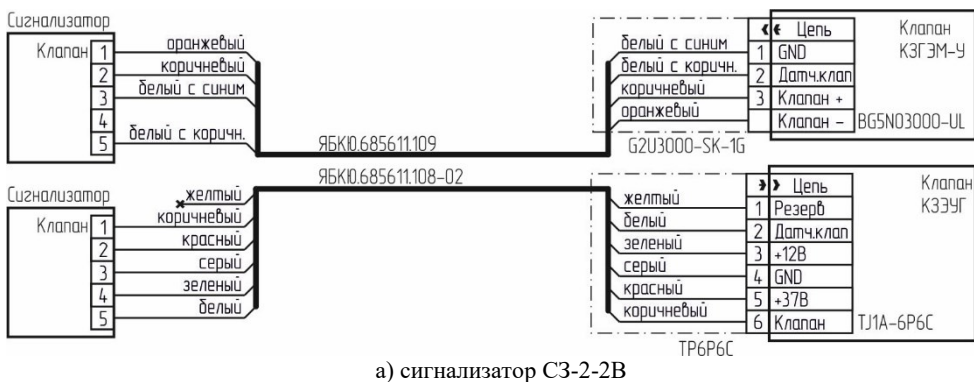
а) сигнализатор СЗ-2-2В
