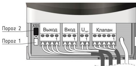
а) сигнализатор С3-2-2В
