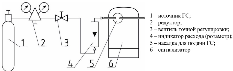
Рисунок Г.1– Схема для настройки порога срабатывания и проверки сигнализатора с применением ГС
