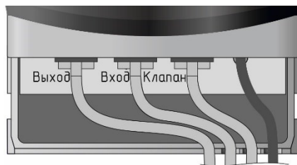
б) сигнализатор С3-2-2ВТ
