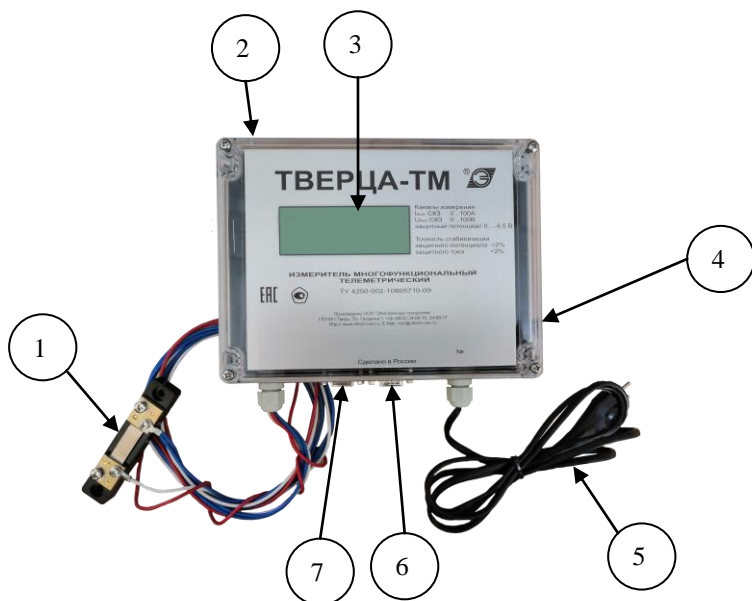
Рис.1 Внешний вид и состав телеметрического модуля «ТВЕРЦА-ТМ» 1. Токоизмерительный шунт (50А, 75mV); 2. разъем SMA для подключения GSM антенны; 3. ЖК индикатор; 4. Вставка плавкая 220В 0,25А; 5. Кабель сетевого питания 220В 6. Измерительно функциональный разъем, 7. Разъем внешних проводных интерфейсов.
