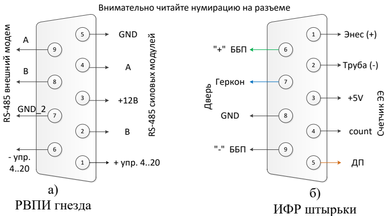
Рис. 3 Назначение контактов разъемов контроллера управления а) – разъем внешних проводных интерфейсов ; б) – измерительно-функциональный
