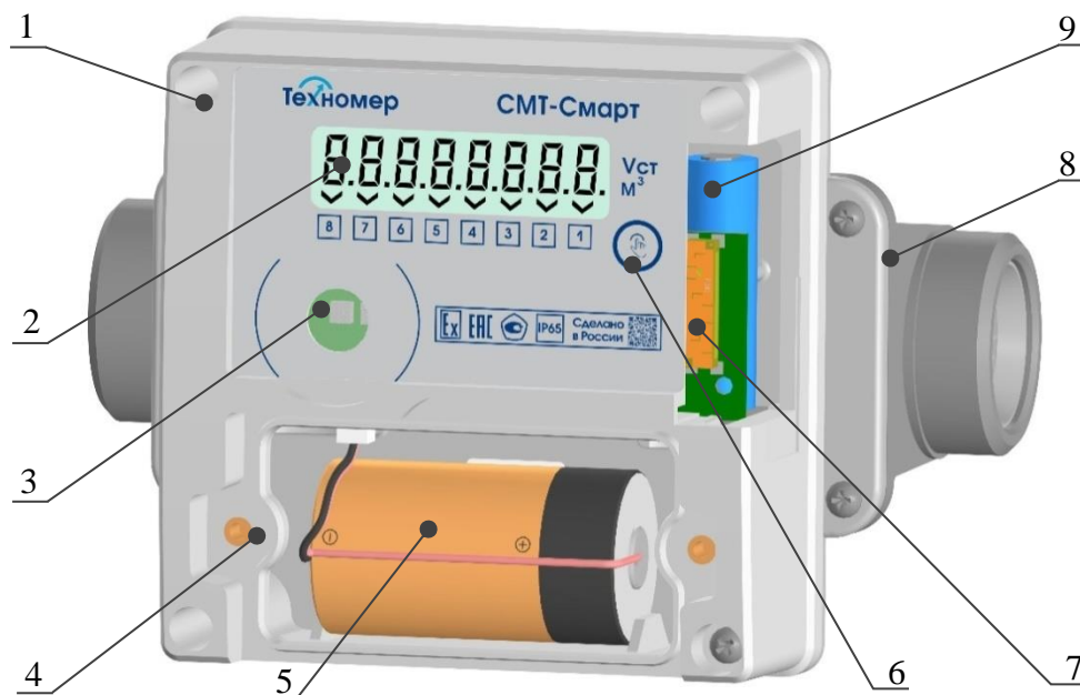
Рисунок 4 – Конструкция СМТ-Смарт
