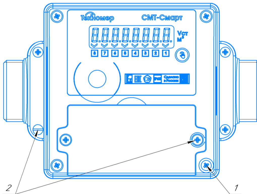
Рисунок 55 – Схема пломбировки СМТ-Смарт
