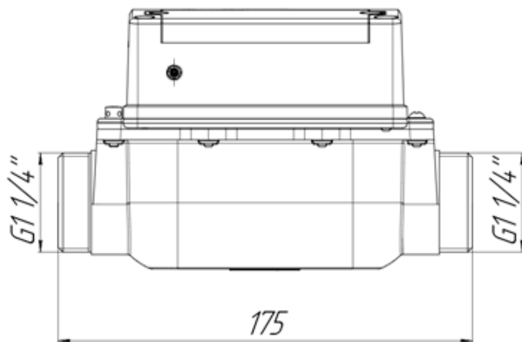
Рисунок А3 – габаритные размеры СМТ-Смарт G4 (G6)-B
