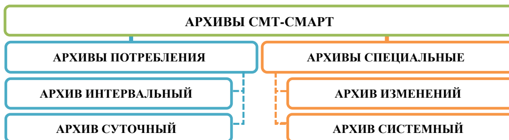
Рисунок 54 – структура архивных данных СМТ-Смарт
