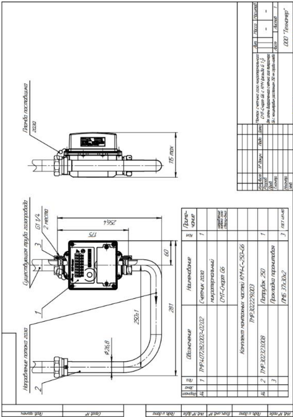
Рисунок Б6 – монтаж СМТ-Смарт Б6 взамен диафрагменного счётчика Г4 с межцентровым расстоянием 250 мм и присоединительными штуцерами резьбой G1 1/4 дюйма.
