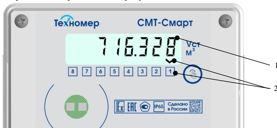
Рисунок 11 – Внешний вид лицевой панели СМТ-Смарт 1 – отображаемые символы, 2 – указатели.
