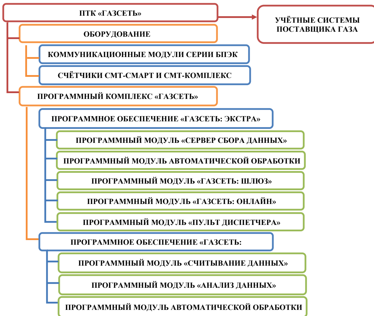
Рисунок В1 – архитектура ПТК «Газсеть»
