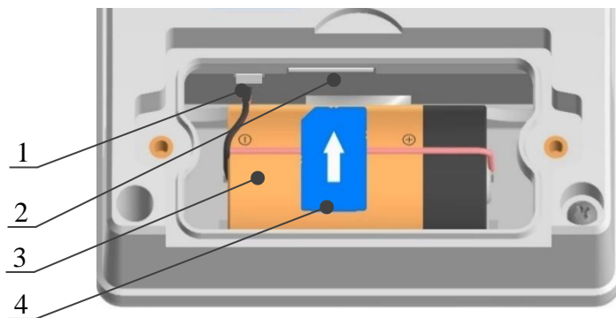
Рисунок 5 – Батарейный отсек СМТ-Смарт
