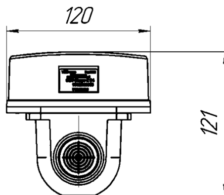
Рисунок А1 – габаритные размеры СМТ-Смарт G4 (G6)
