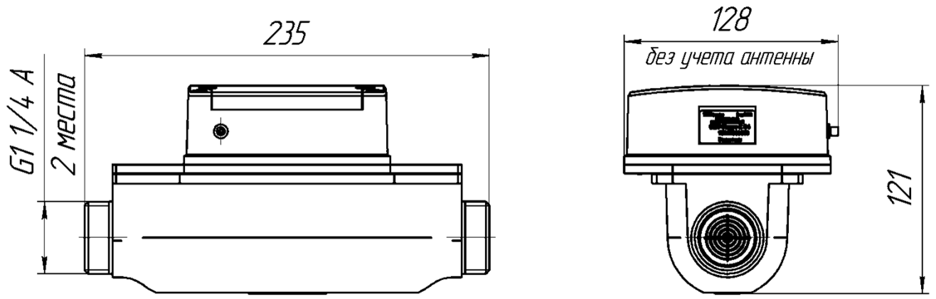
Рисунок А4 – габаритные размеры СМТ-Смарт G10-В
