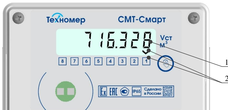
Рисунок 6 – Внешний вид лицевой панели СМТ-Смарт 1 – отображаемые символы, 2 – указатели.
