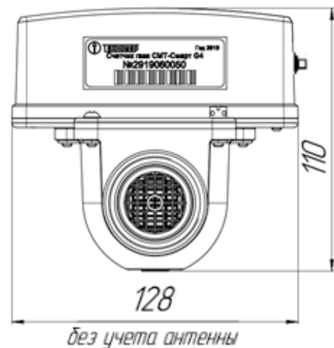
Рисунок А3 – габаритные размеры СМТ-Смарт G4 (G6)-B
