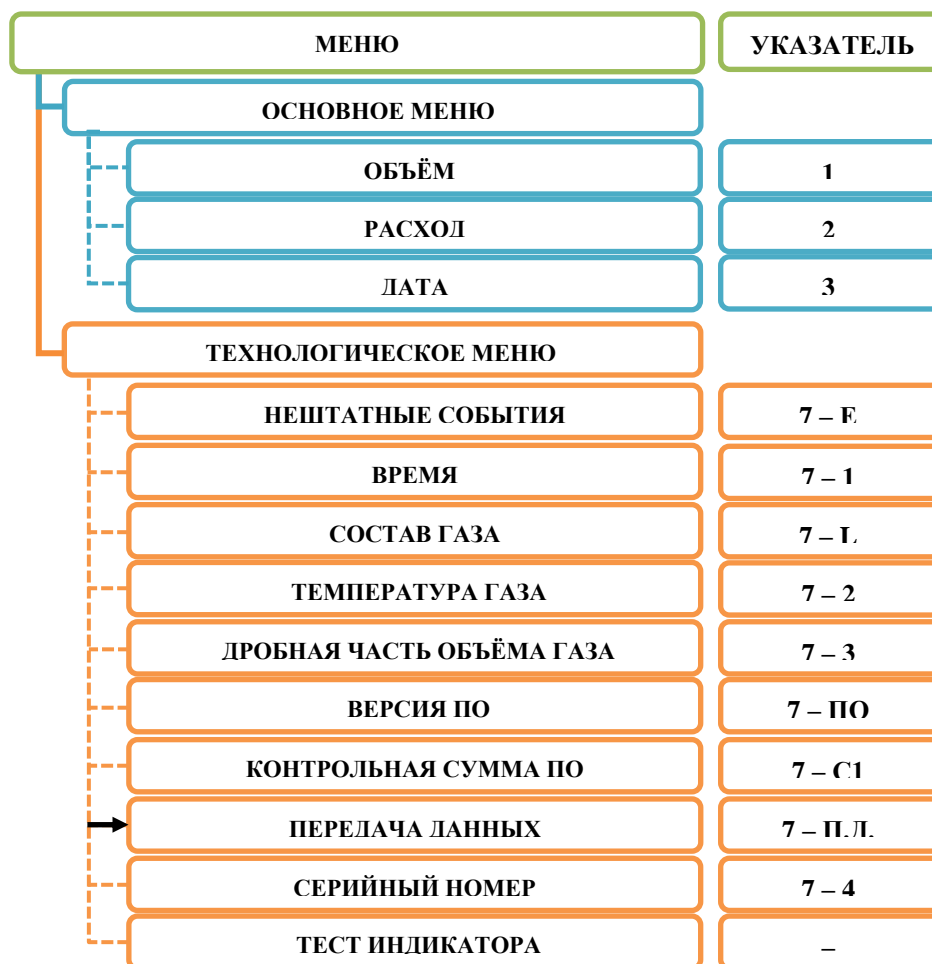
Рисунок 7 – Структура меню
