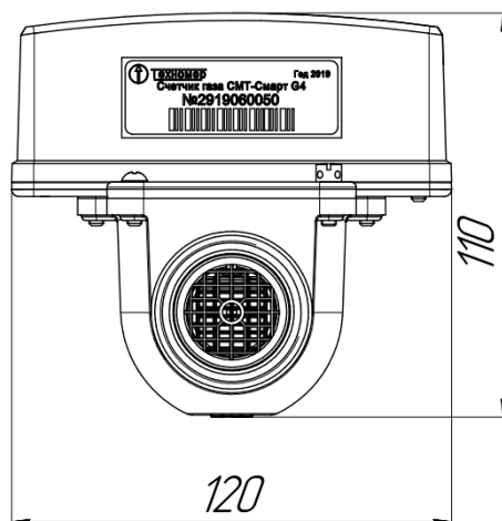
Рисунок А1 – габаритные размеры СМТ-Смарт G4 (G6)
