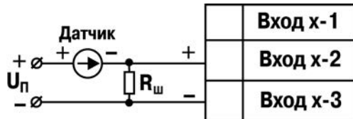
Рисунок Б.11 – Схема подключения активного датчика с токовым выходом 0...5 мА или 0(4)...20 мА R_{ш}=50,000 \pm 0,025 \text{ Ом}
