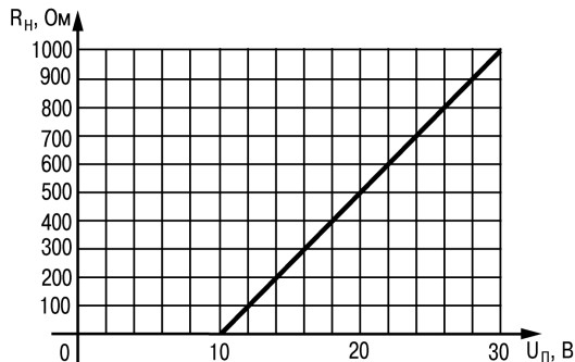
Рисунок 3.18 – График зависимости R_H(U_{п})
