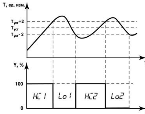
Рисунок Ж.1 – АНР прибора, работающего в режиме нагревателя
