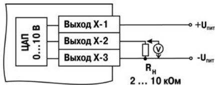
Рисунок Б.7 – Схема подключения нагрузки к ВУ типа У
