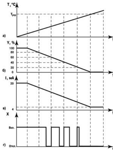
Рисунок 3.11 – Принцип управления в режиме «Нагреватель»:
