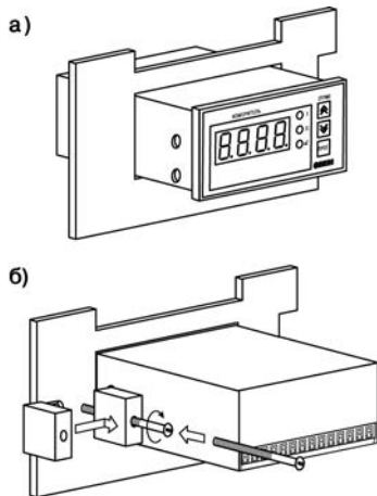
Рисунок 5.1 - Монтаж прибора щитового крепления
