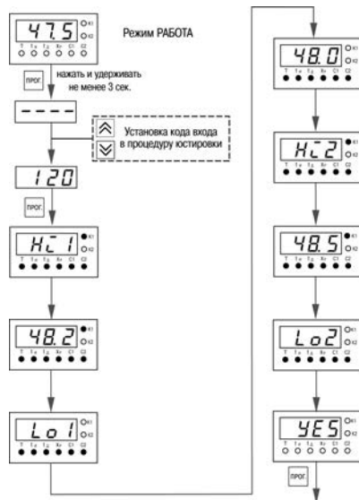
Рисунок Ж.2 – Последовательность запуска индикации АНР для ТРМ10-Щ1.Р
