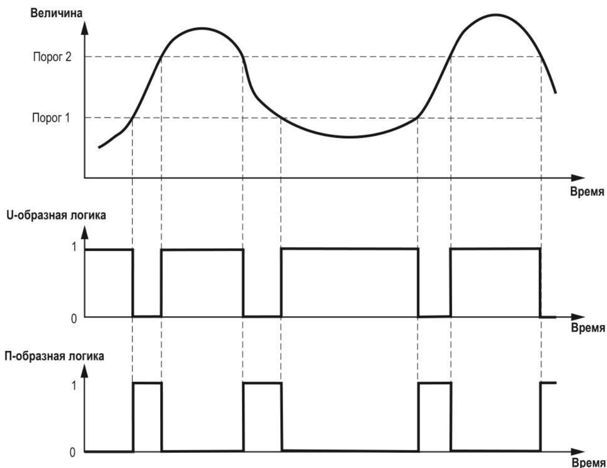
Рисунок 9.53 – Работа Инспектора по U-образной и П-логикам
