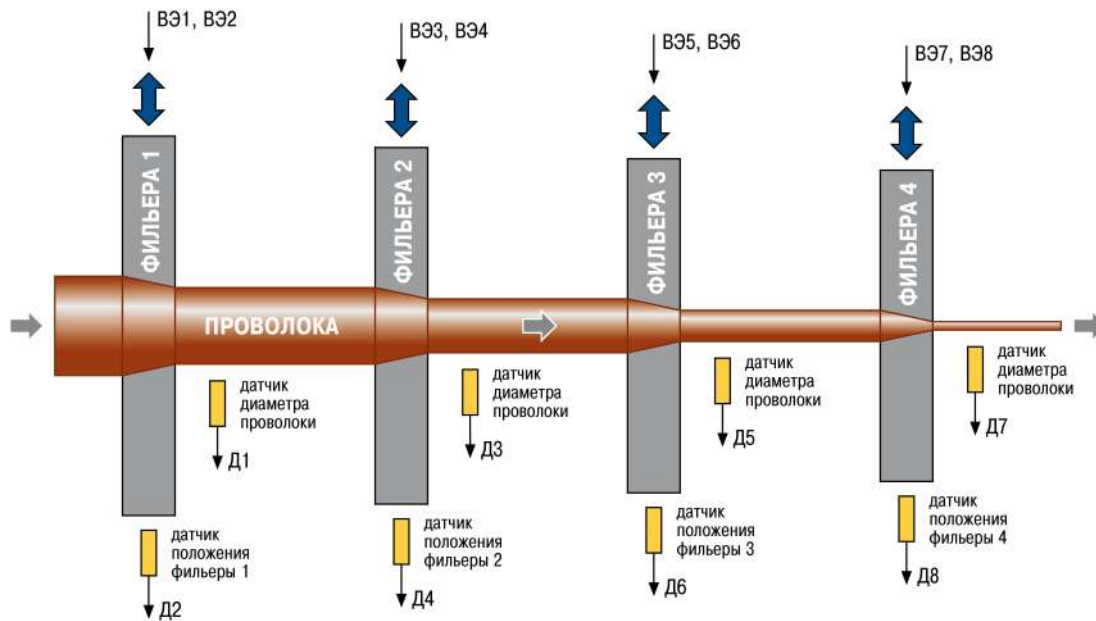
Рисунок 7.8 – Использование 8-канального регулятора ТРМ148 3-ей модификации в управляемой автоматизированной системе из четырех фильер для получения проволоки
