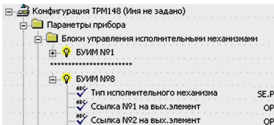
Рисунок 9.34 – Конфигуратор. Настройка БУИМ
