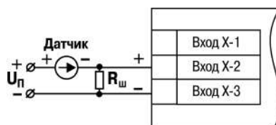
Рисунок 5.8 – Схема подключения пассивного датчика с токовым выходом 0...5,0 мА или 0(4)...20 мА R_{ш}=100,000 \pm 0,025 Ом
