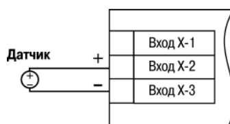
Рисунок 5.7 – Схема подключения активного датчика с выходом в виде напряжения -50...50 мВ или 0...1 В
