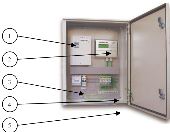
Рисунок 1. Внешний вид и состав комплекса телеметрии ГРП.
