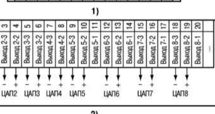
Рисунок 19 – Схема подключения твердотельных реле прибора: 1) в корпусе Щ4, 2) в корпусе Щ7
