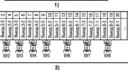
Рисунок 17 – Схема подключения симисторных оптопар прибора: 1) в корпусе Щ4, 2) в корпусе Щ7
