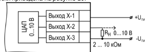
Рисунок 20 – Схема подключения нагрузки к ВУ типа У
