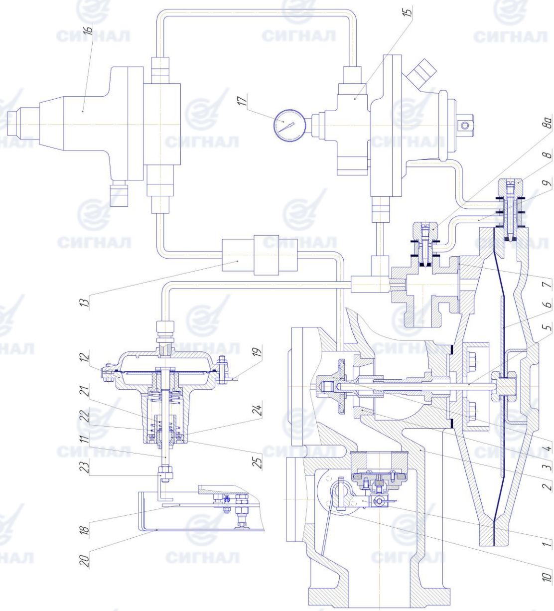
1-клапан отсеchnой; 2-исполнительное устройство; 3-седло; 4-клапан рабочий; 5-стержень; 6-мембрана исполнительного устройства; 7-дрoссельная шайба; 8, 8а-дрoссели регулируемые; 9-пружина импульсная входного газопровода; 10-пружина отсеchnого клапана; 11-шток механизма контроля; 12-механизм контроля; 13-фильтр; 15-регулятор управления (КН-2); 16-стабилизатор; 17-манометр; 18-рычаг отсеchnого клапана; 19-кронштейн; 20-кожух; 21-пружина малой; 22-пружина большой; 23-скоба; 24-рег. винт малой пружины; 25-рег. винт большой пружины.
